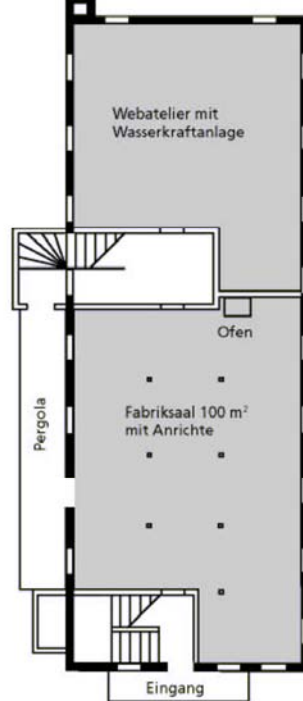
2. Geschoss
